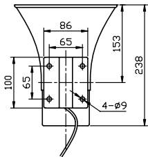
安装尺寸图 (单位: mm)
