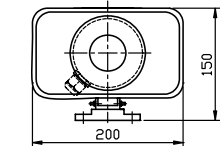
BC-3A 带接线盒
